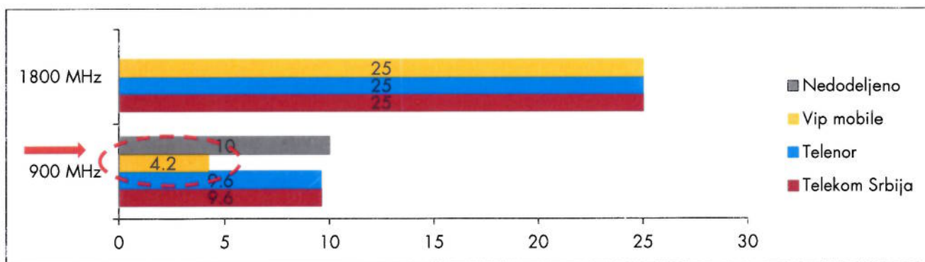
Slika 2: Raspodela frekvencija između operatora na osnovu nacrtu Pravilnika od 18.08.2014.
